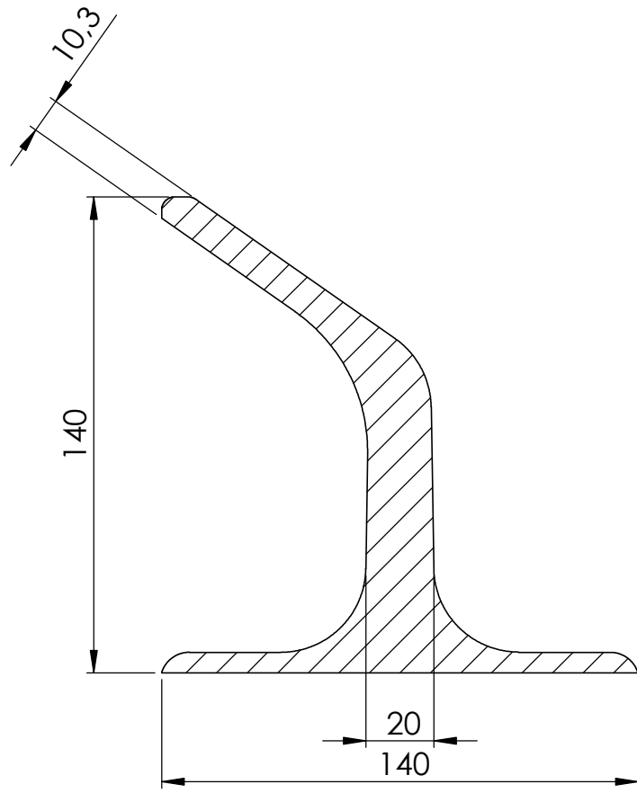
SEZIONE C-C
